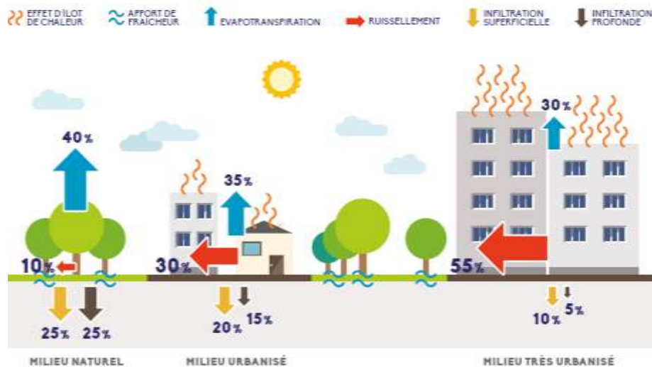
Illustration de l'impact de l'imperméabilisation sur le cycle de l'eau
